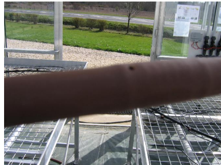
Goutteurs autorégulant intégrés dans le tuyau avec filtre
